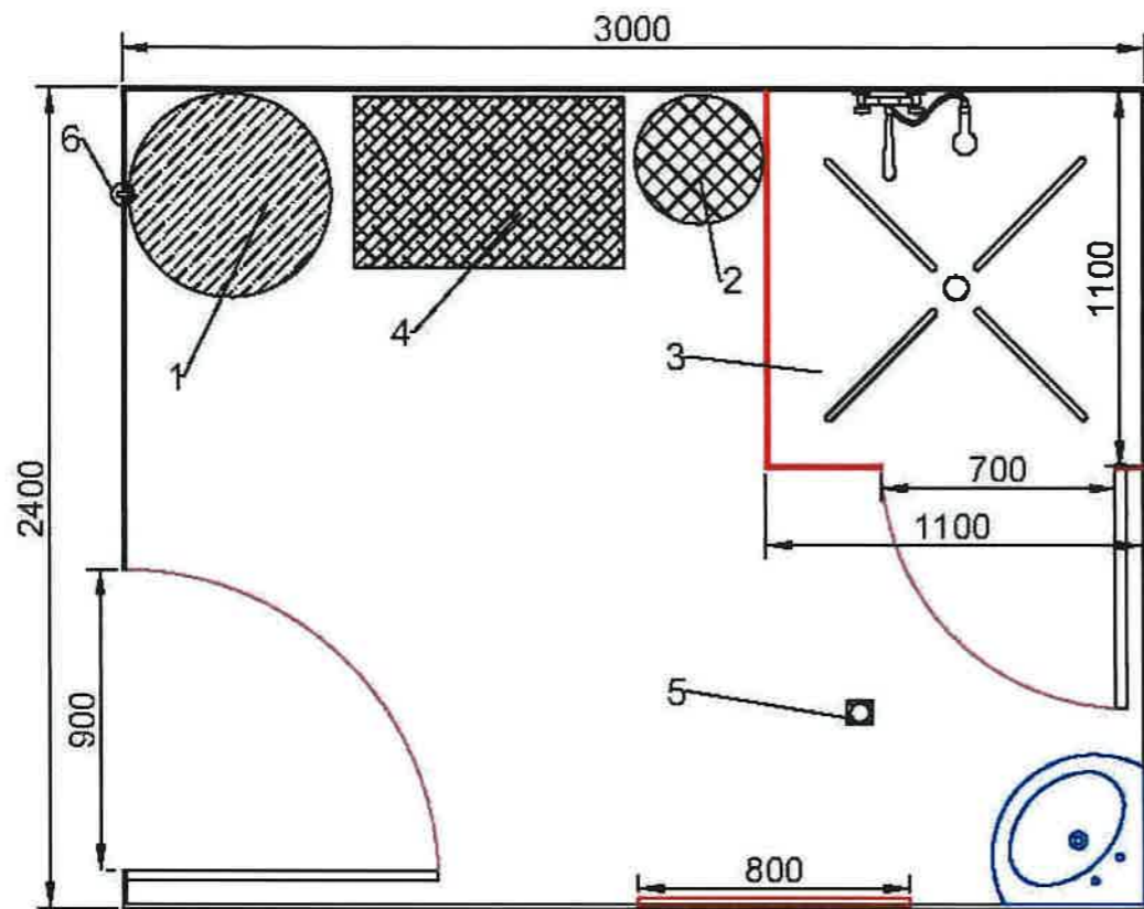
План душевого блока.
